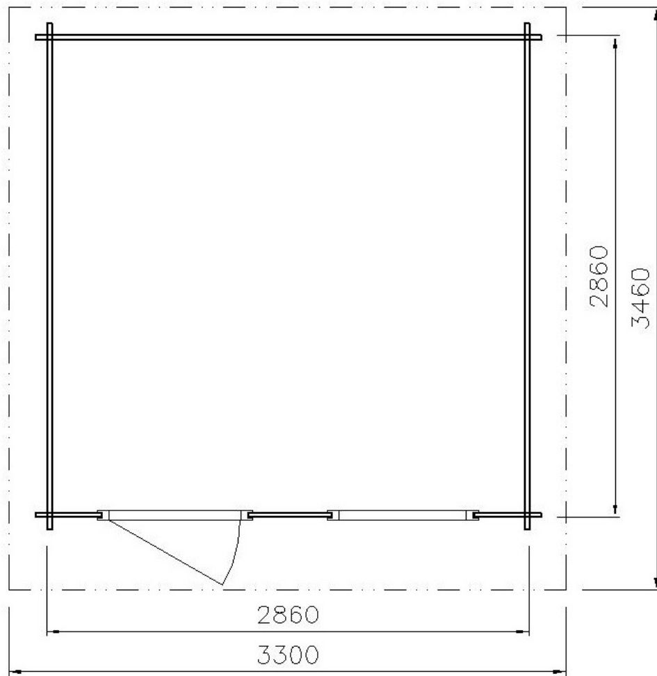
PŮDORYS
