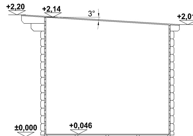
ŘEZ
