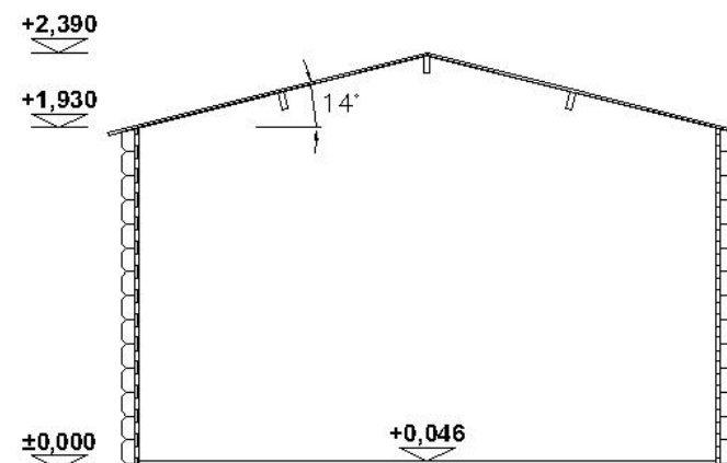
ŘEZ
