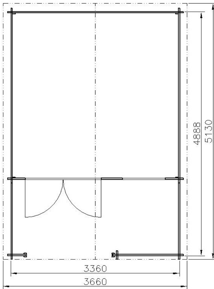
PŮDORYS
