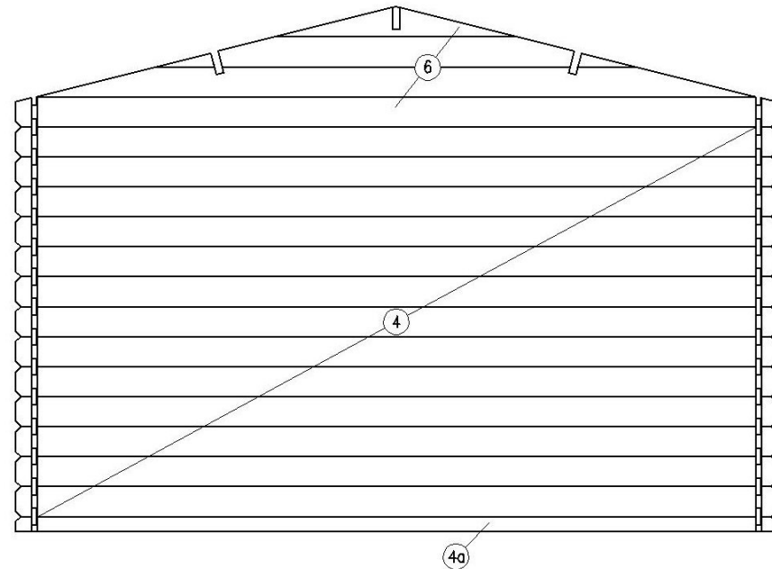
ZADNÍ STĚNA D
