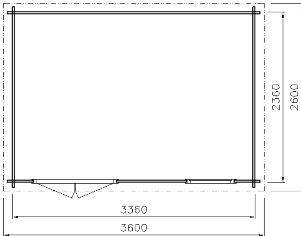
PŮDORYS
