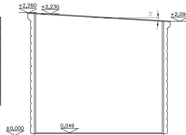
ŘEZ
