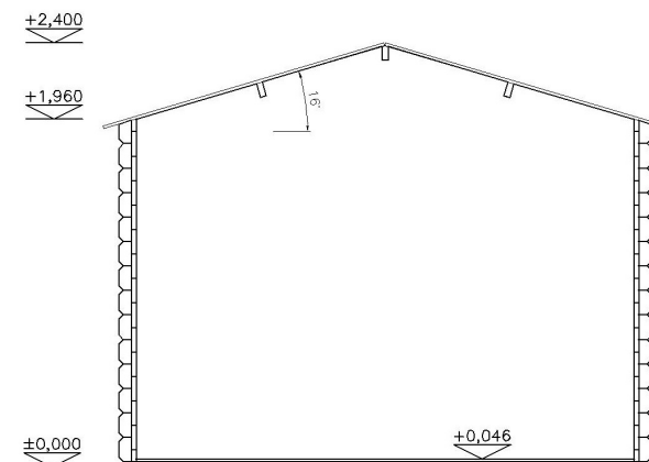
ŘEZ
