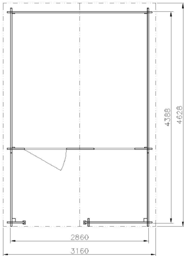
PŮDORYS
