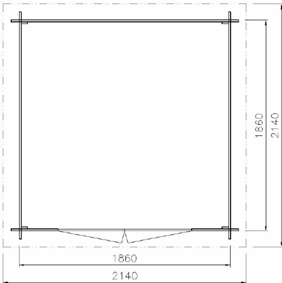
PŮDORYS
