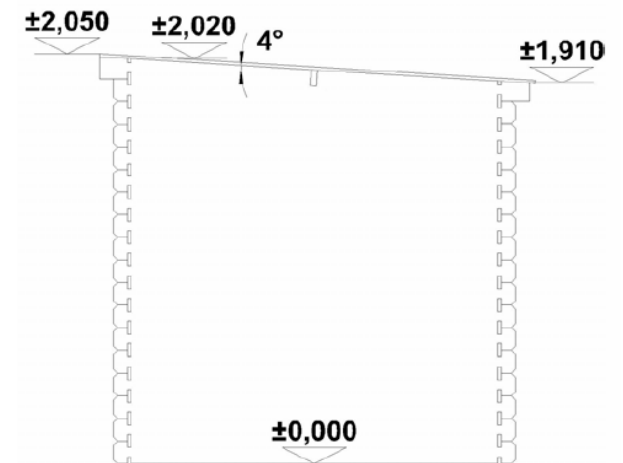
ŘEZ
