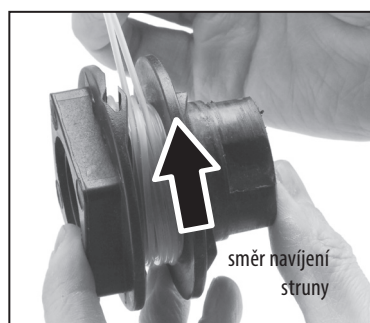
Obr.10, navíjení struny na cívku
