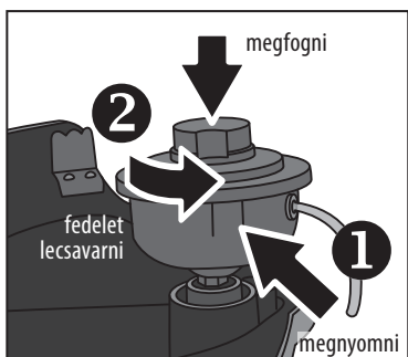
8. ábra. A tekercs levétele a menesztőről.
