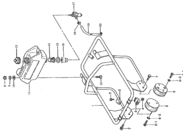
OCHRANNÝ RÁM
